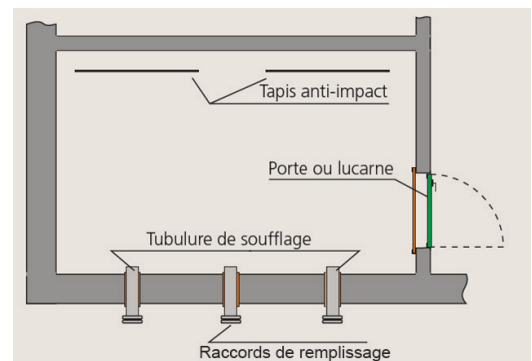
Schéma de silo dont la largeur est supérieure à 2,2 mètres (Source : propellet.ch)
