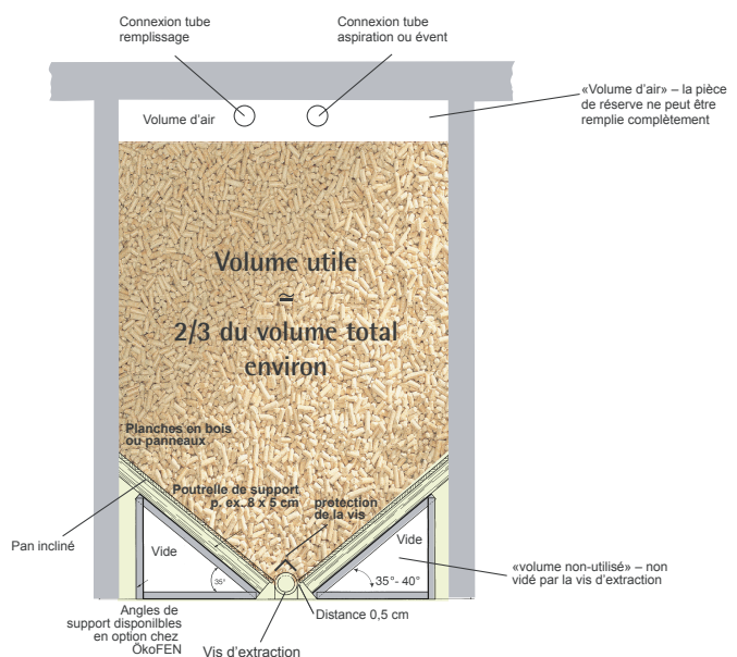
Coupe d'une pièce de réserve standard
