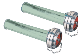
2 raccords de remplissage (réf. ZK100FB) et tuyaux de remplissage standards (réf. ZR050)
