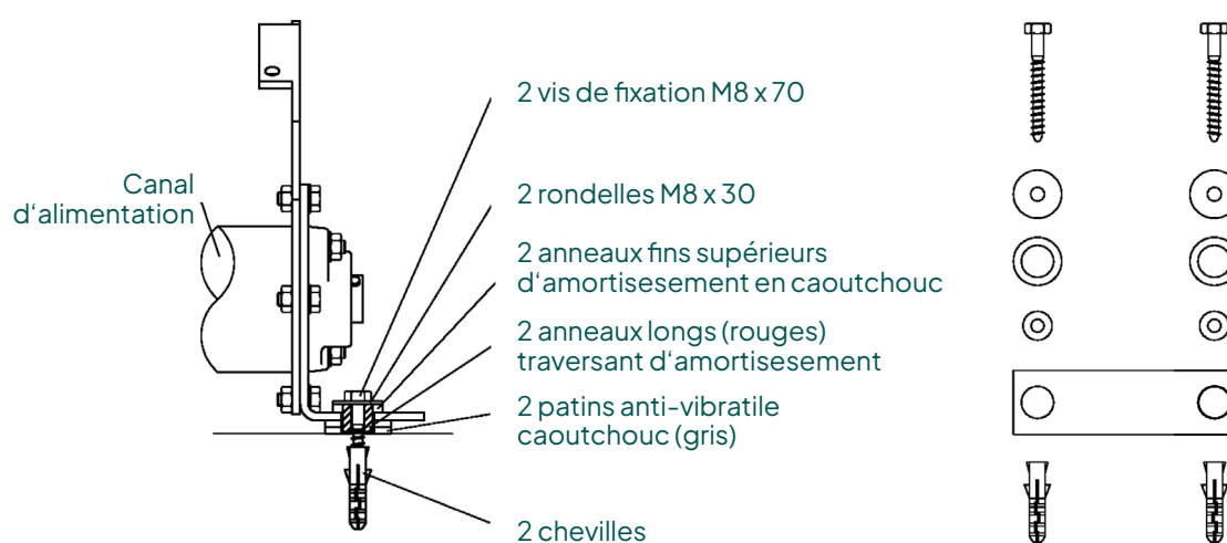
Détail du palier de vis d'extraction
