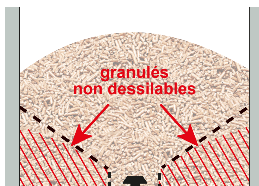
sans pan incliné : plus de granulés stockés mais pas déssilés
