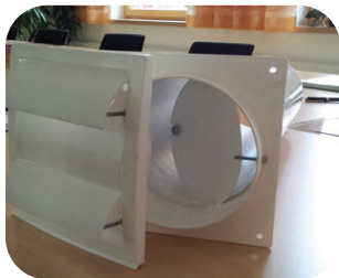
Tuyau PVC d'aération avec volets et clapet anti-retour d'air (réf. Z135 – ouverture effective de 176 cm²)
