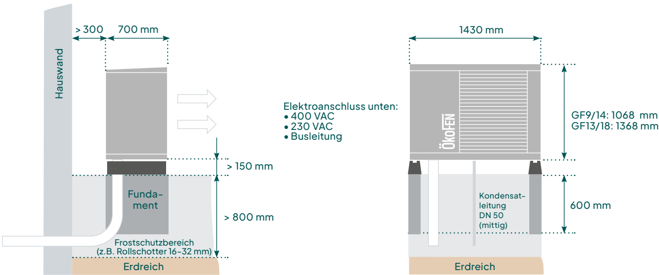
Aufstellungsskizze: Detaillierter Fundamentplan in den Planungsunterlagen.
