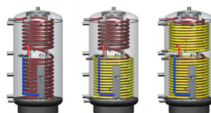
Systemspeicher mit Edelstahlwellrohr-Wärmetauscher und ohne, mit 1 oder 2 Solarregistern
