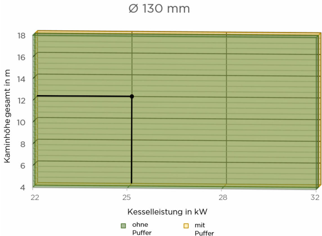
Abb. 3: Maximal zulässige Kaminhöhe bei gegebener Kesselleistung
