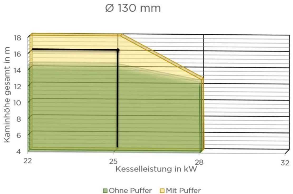
Abb. 5: Maximal zulässige Kaminhöhe bei gegebener Kesselleistung
